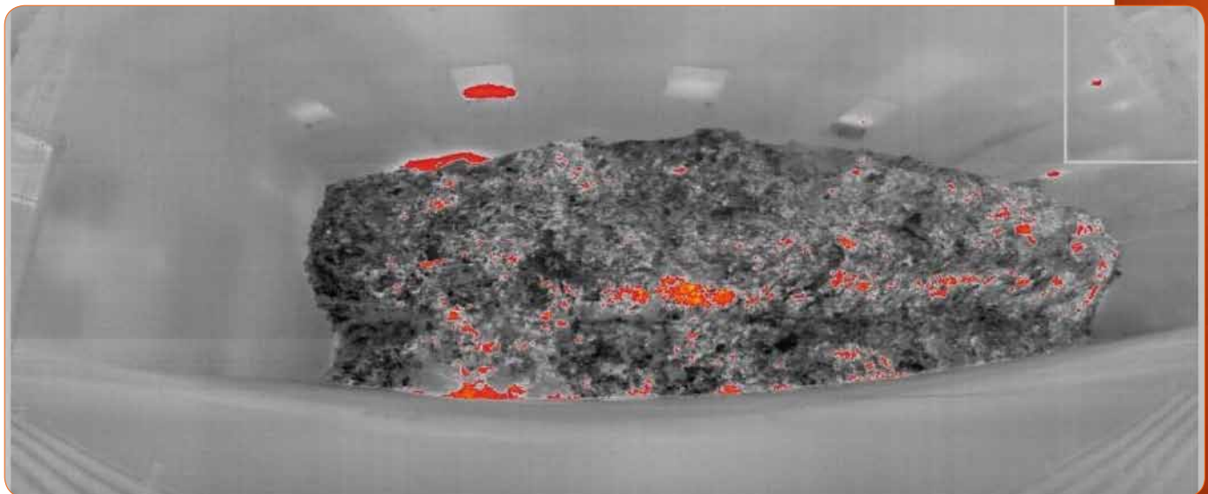
Panoramathermografie: Ansicht eines Müllbunkers mit der patentierten abrioVision® Software
